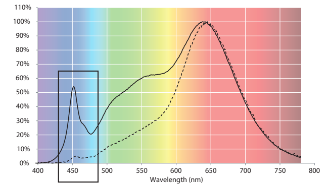
Lichtspektrum: — bei Volllicht mit 2700–3000 K ----- bei minimaler Helligkeit mit 1800 K
