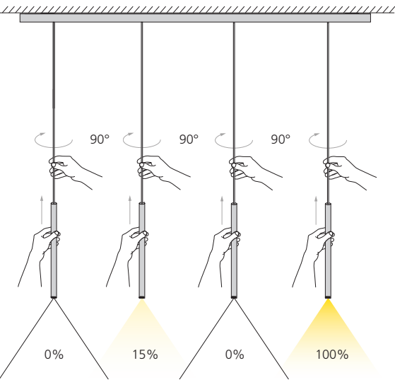
Axiales Drehen von Pendel = Ein / Aus, zwei Helligkeitsstufen (100% oder 15%)
